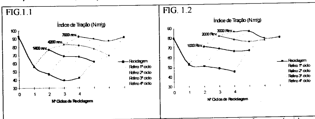
FIGURA 1: Índice de Tração em função dos ciclos de reciclagem com aplicação de refino em cada ciclo para recuperação da propriedade. (Fig. 1.1- Pinus ; Fig. 1.2- Eucalipto).
