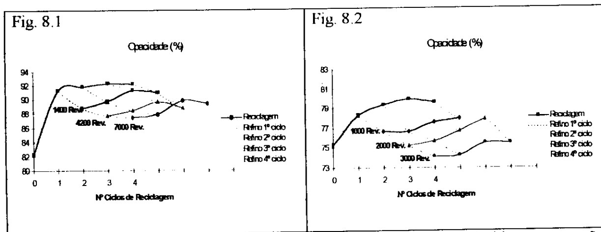
FIGURA 8: Opacidade em função dos ciclos de reciclagem com aplicação de refino em cada ciclo para recuperação da propriedade. (Fig. 8.1- Pinus ; Fig. 8.2- Eucalypto).
