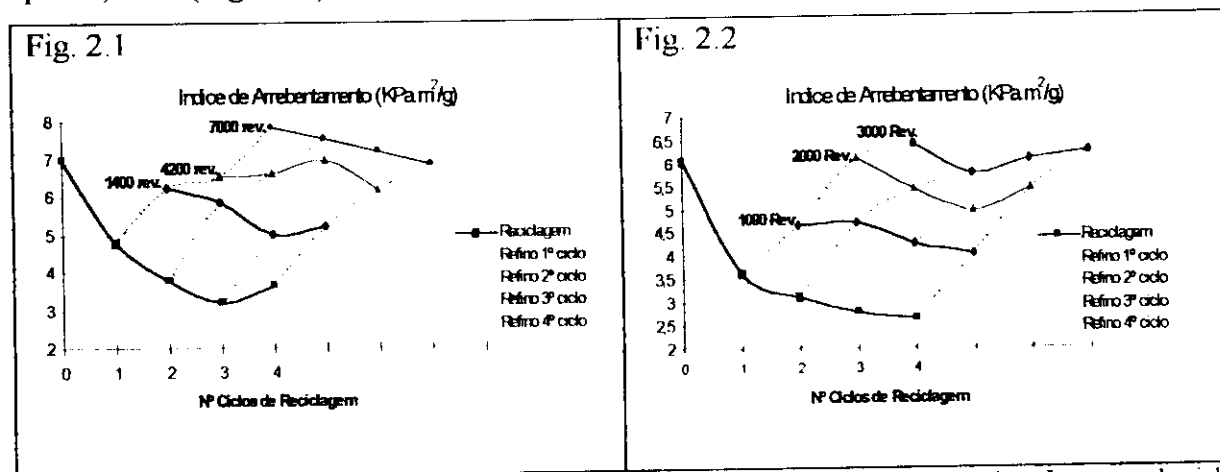
FIGURA 2: Índice de Arrebentamento em função dos ciclos de reciclagem com aplicação de refino em cada ciclo para recuperação da propriedade. (Fig. 2.1- Pinus ; Fig. 2.2- Eucalipto).
