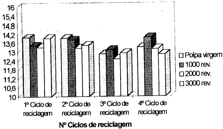
Figura 10: Viscosidades da polpa de Eucalipto em cada ciclo de reciclagem e aos níveis de refino utilizado para recuperação de propriedades. Figure 10: Viscosity of Eucalyptus pulp in function of the recycling cycles and each refine levels.
