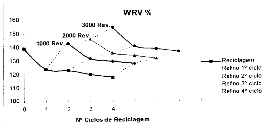
Figura 11: WRV - Índice de Retenção de Água para a polpa de Eucalypto em função dos ciclos de reciclagem e aos níveis de refino.
