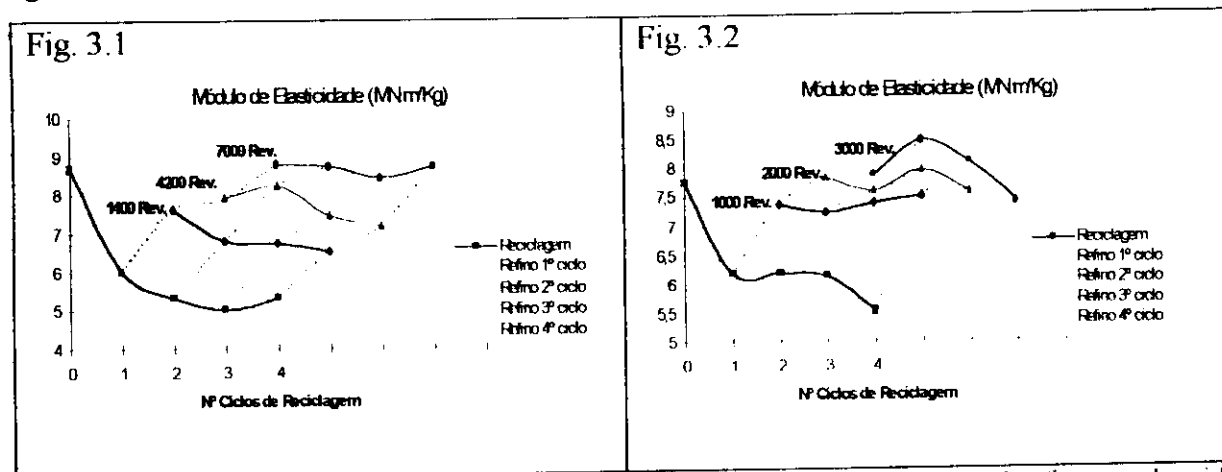
FIGURA 3: Módulo de Elasticidade Específico em função dos ciclos de reciclagem com aplicação de refino em cada ciclo para recuperação da propriedade. (Fig. 3.1- Pinus ; Fig. 3.2- Eucalipto).
