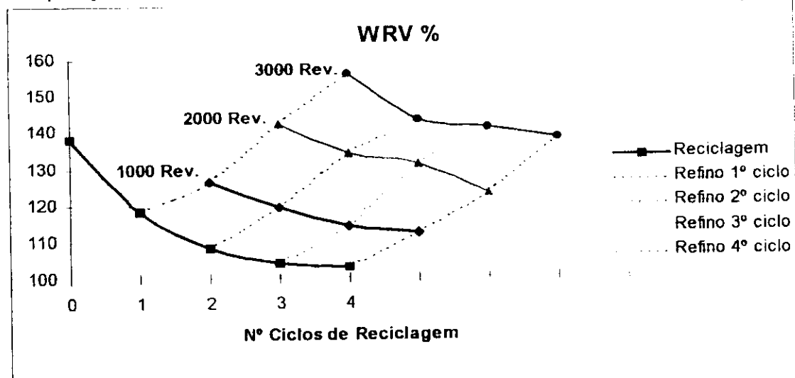
Figura 12: WRV - Índice de Retenção de Água para polpa de Pinus em função dos ciclos de reciclagem e aos níveis de refino.
