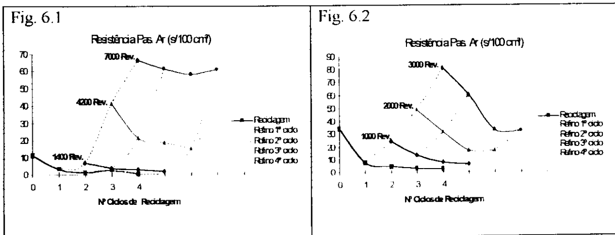
FIGURA 6: Resistência à Passagem Ar em função dos ciclos de reciclagem com aplicação de refino em cada ciclo para recuperação da propriedade. (Fig. 6.1- Pinus ; Fig. 6.2- Eucalipto).
