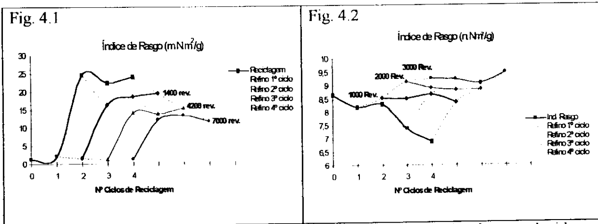
FIGURA 4: Índice de Rasgo em função dos ciclos de reciclagem com aplicação de refino em cada ciclo para recuperação da propriedade. (Fig. 4.1- Pinus ; Fig. 4.2- Eucalipto).
