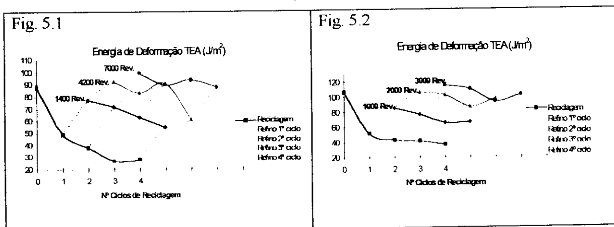
FIGURA 5: Energia de Deformação em função dos ciclos de reciclagem com aplicação de refino em cada ciclo para recuperação da propriedade. (Fig. 5.1- Pinus ;Fig. 5.2- Eucalipto).
