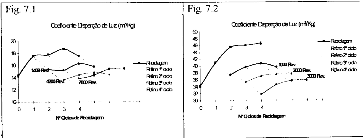
FIGURA 7: Coeficiente Disp. Luz em função dos ciclos de reciclagem com aplicação de refino em cada ciclo para recuperação da propriedade. (Fig. 7.1- Pinus ; Fig. 7.2- Eucalypto).
