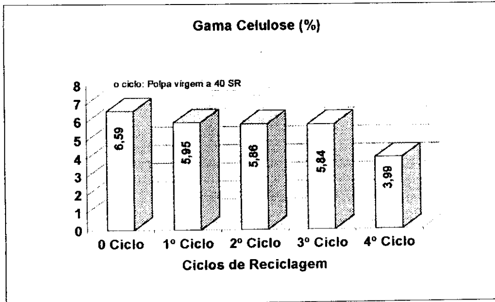
Figura 9- Teor de \gamma celulose na polpa reciclada de Eucalipto. Figure 9- \gamma cellulose content in recycled pulp of Eucalyptus.
